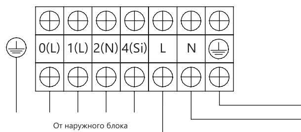
Клеммный терминал наружного блока
